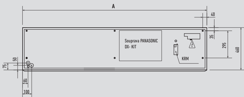
Pohled shora
