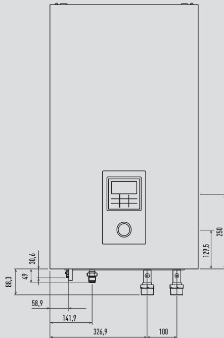
Čelní pohled
