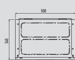
Pohled shora
