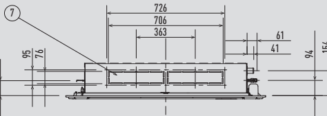
Čelní pohled
