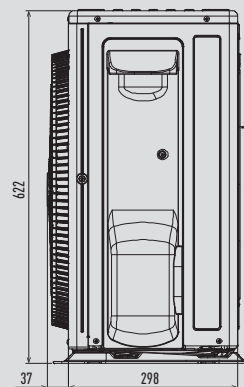
Boční pohled
