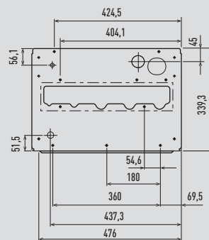
Spodní pohled
