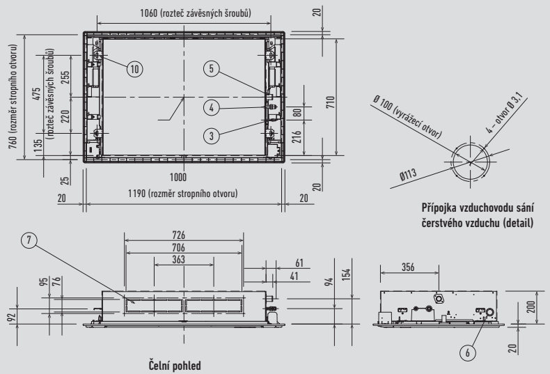
Čelní pohled
