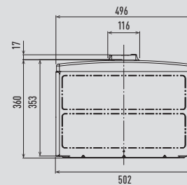
Pohled shora
