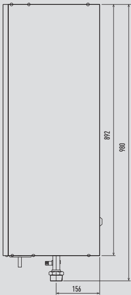
Boční pohled
