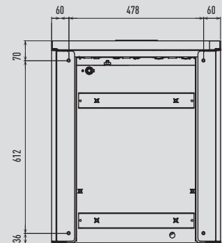
Spodní pohled
